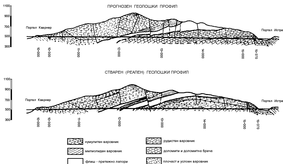
слика 4-4 Пројнозен и стварен геолошки профил (тунел Учка - Хрватска)
