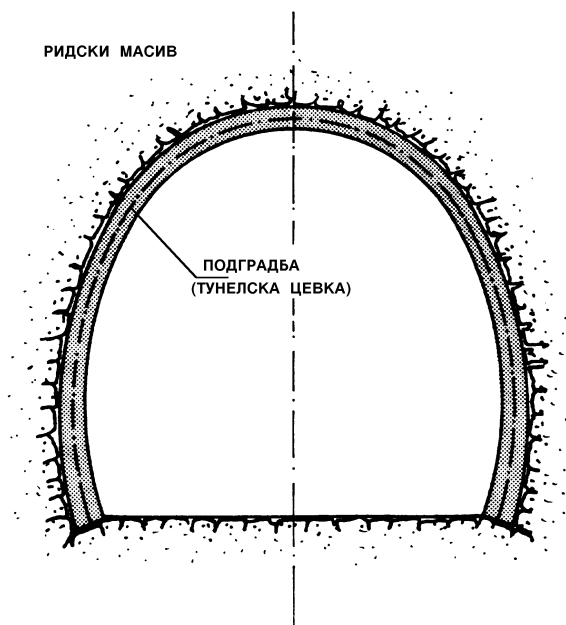
слика 4-3 - Најречен пресек на тунел
