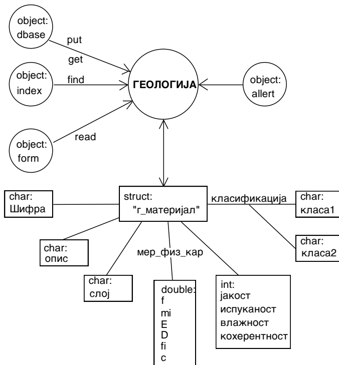
Слика 4-10 Атрибути на објектот "Геологија"
