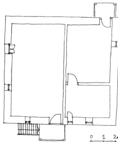
Сл.2. Основа на куќа на приземје и вкопан подрум, с.Цер, 19 ти век
