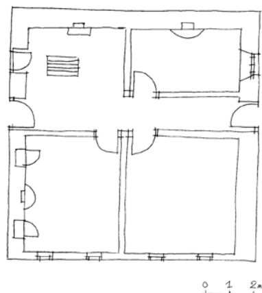
Сл.1. Основи на амбар во две нивоа, с.Раветино, 19ти век
