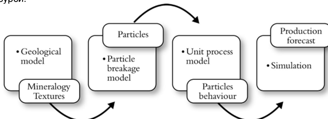
Слика 2. Геметаллуршкиот концепт базиран на честички, модифициран од Ламберг (2011). Минералогски модел и текстури го поврзуваат геолошкиот модел и процесниот модел. Во процесот на модел минерали се третираат како честички. Од минералните информации, присуството на честички се генерира преку модел на кршење на честички
