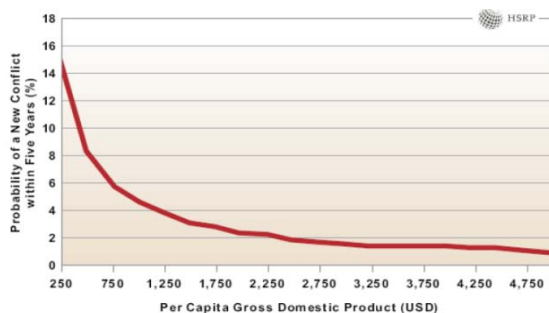
Слика 6. Бруто домашниот производ (GDP-БДП) по глава на жител во сооднос со можниот ризик од вооружен конфликт.
