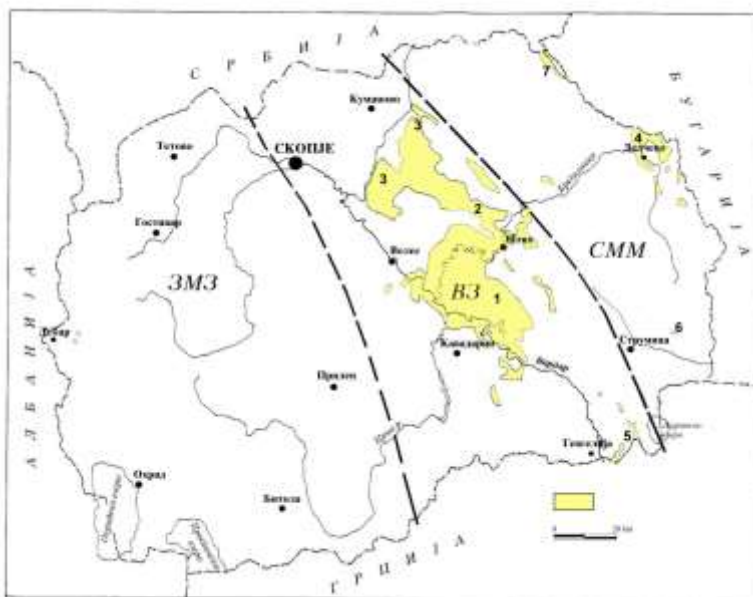
Слика 1 - Распространение на палеогените седименти во Македонија 1 - Тиквешки басен, 2 - Овчеполски басен, 3 - Скопско-Кумановски басен, 4 - Делчевски басен, 5 - Гевгелиско-Валандовски басен, 6 - Струмички басен, 7 - Деве Баирски басен
