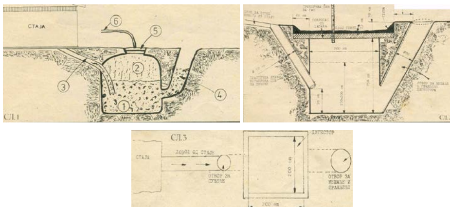
Slika 2: Kineski biodigestor
