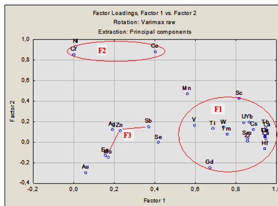
Fig. 1 Loading plots of F1 and F2
