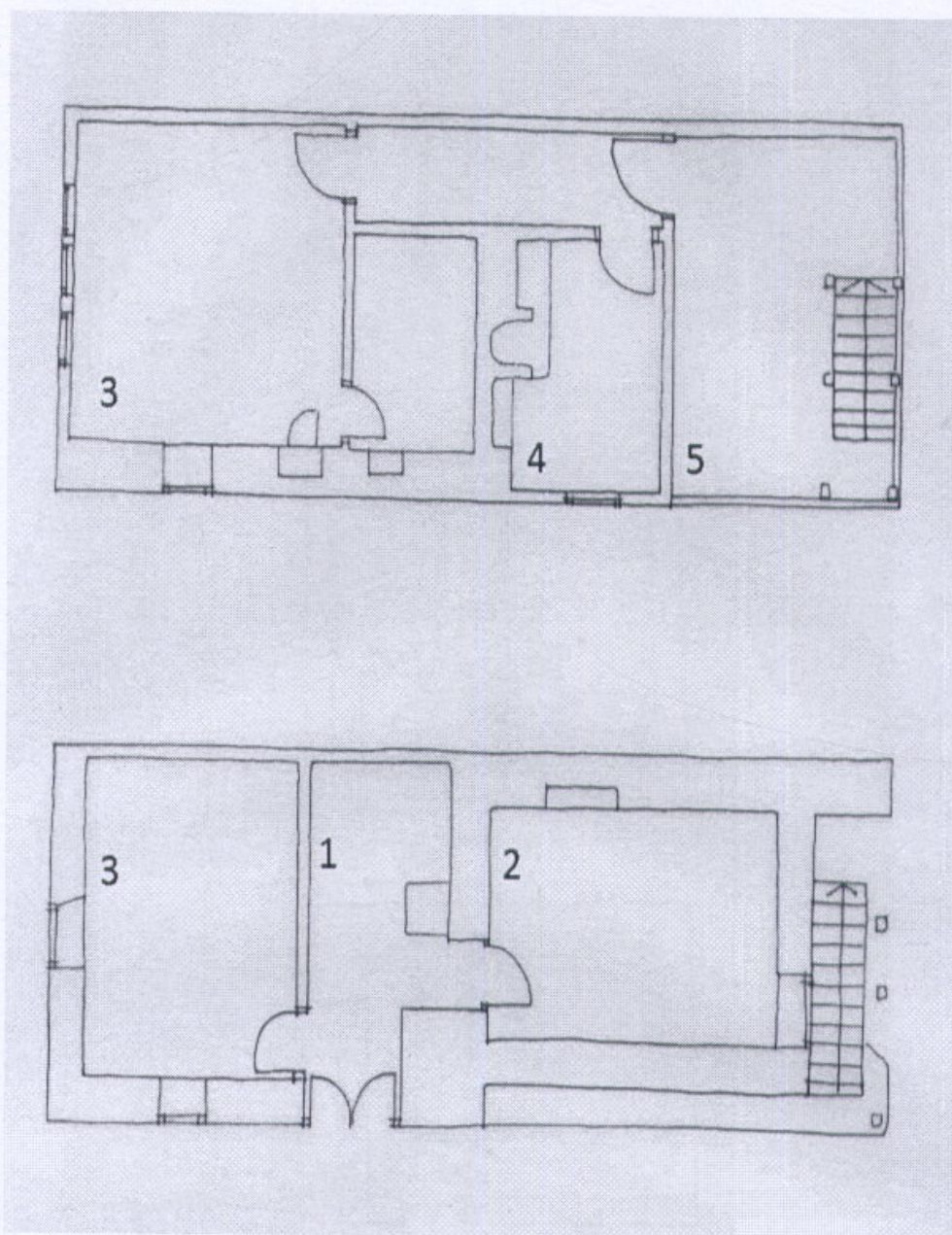
цр. 3. основи на куќа во две нивоа, со асиметричен распоред на просториите (1. трем; 2. земник; 3. одаја; 4. куќа - кујна; 5. чардак)
