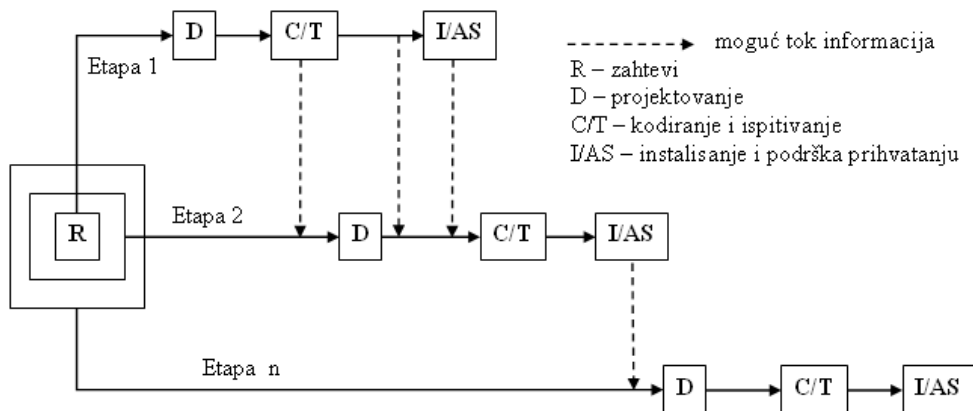
Slika 3. Inkrementalni model [4]
